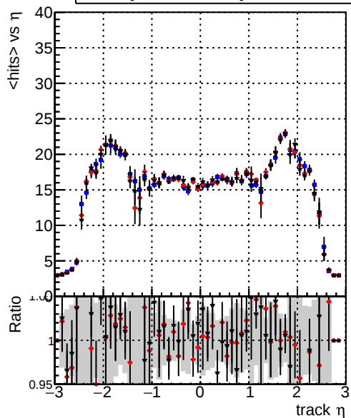
mean hits — DQM_TT_CKF_ORIG — DQM_TT_CKFlowPtQ_ORIG — DQM_TT_CKFlowPtQ_MODIF
