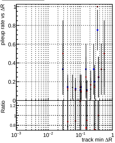
Legend: DQM TT CKF ORIG (blue), DQM TT CKFLowPtQ ORIG (red), DQM TT CKFLowPtQ MODIF (black)
