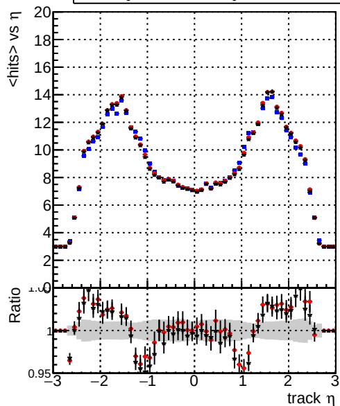
mean hits vs \eta DQM_TT_CKF_ORIG DQM_TT_CKFLowPtQ_ORIG DQM_TT_CKFLowPtQ_MODIF
