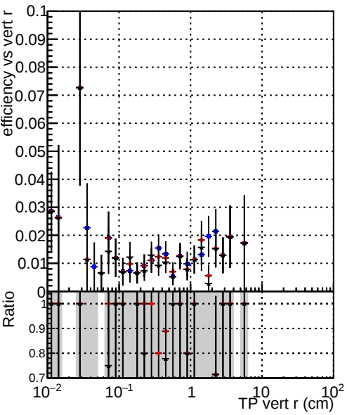
Efficiency vs vertpos DQM_TT_CKF_ORIG DQM_TT_CKFLowPtQ_ORIG DQM_TT_CKFLowPtQ_MODIF
