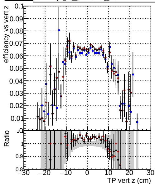
Efficiency — DQM_TT_CKF_ORIG — DQM_TT_CKFLowPtQ_ORIG — DQM_TT_CKFLowPtQ_MODIF
