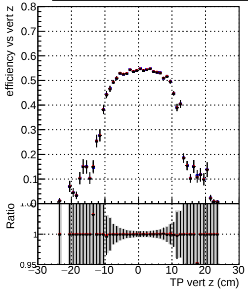
Efficiency vs. sim PV z —●— DQM_TT_CKF_ORIG —●— DQM_TT_CKFLowPtQ_ORIG —●— DQM_TT_CKFLowPtQ_MODIF
