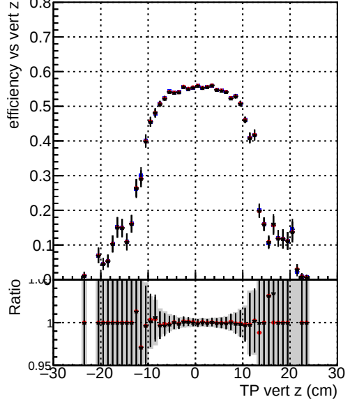
Efficiency vs. TP vert z (cm) Legend: - DQM_TT_CKF_ORIG (blue circles) - DQM_TT_CKFlowPtQ_ORIG (red circles) - DQM_TT_CKFlowPtQ_MODIF (black circles)
