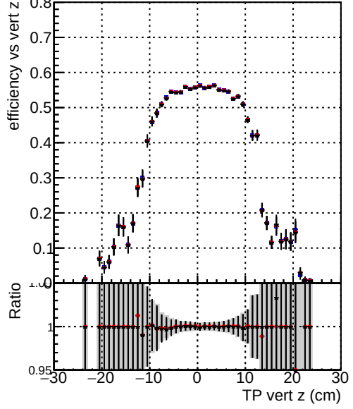
Efficiency vs. TP vert z (cm) — DQM_TT_CKF_ORIG — DQM_TT_CKFlowPtQ_ORIG — DQM_TT_CKFlowPtQ_MODIF
