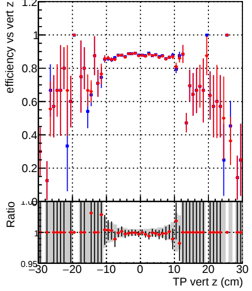
Efficiency vs. TP vert z — DQM_7571_noSel — DQM_7572_noSelS
