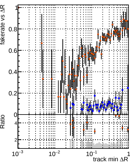
Fake rate vs \Delta R(\text{track, jet}) Legend: DOM CKE Ttbar DOM mktfit Ttbar DOM mktfit Ttbar PU DOM mktfit Ttbar PU - BNN DOM mktfit Ttbar PU - BNN 100 DOM mktfit Ttbar PU - BNN 1000
