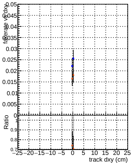
DOM GKE TTher DOM mREIL TTherPU-DNN DOM mREIL TTherPU-DNN-100
