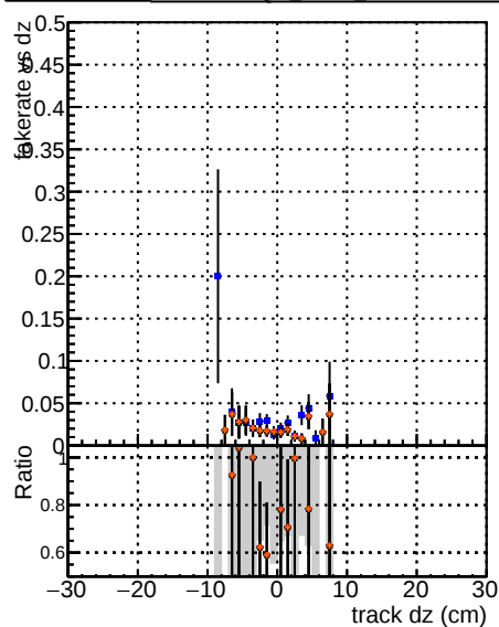
DOM GKE TTher DOM mREIL TTherPU-DNN DOM mREIL TTherPU-DNN-100
