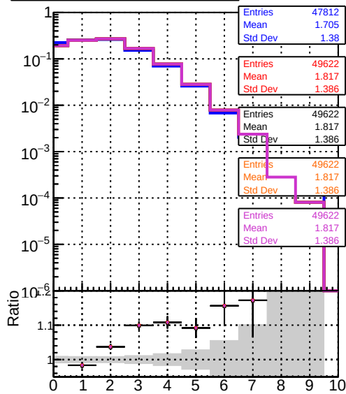
DOM CKE Ttbar DOM mkFit TtbarPU-updated DOM mkFit TtbarPU-updated-newPLDNN DOM mkFit TtbarPU-updated-newPLDNN-2 DOM mkFit TtbarPU-updated-DNNsgcd13
