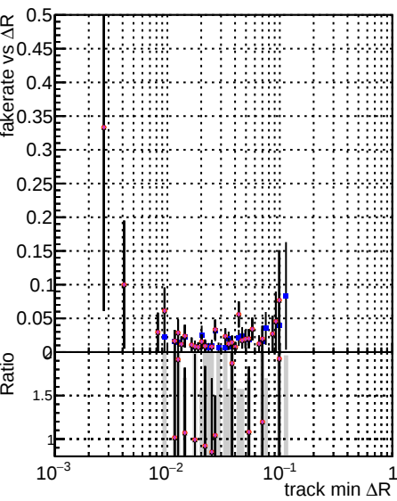
Fake rate vs \Delta R(\text{track, jet}) DQM CKF Tthor PU-updated newPLDNN_2 DQM CKF Tthor PU-updated newPLDNN_2 DQM CKF Tthor PU-updated newPLDNN_2
