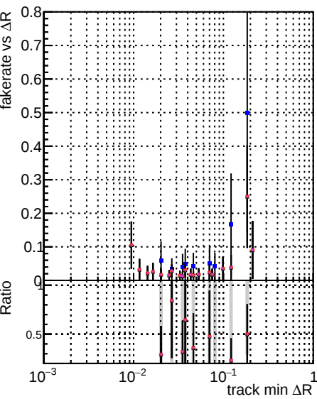
Fake rate vs \Delta R(\text{track, jet}) DQM CKE TThor DQM+PU DQM+PU+updated newPLDNN_2 DQM+PU+updated+DNNsqcd13
