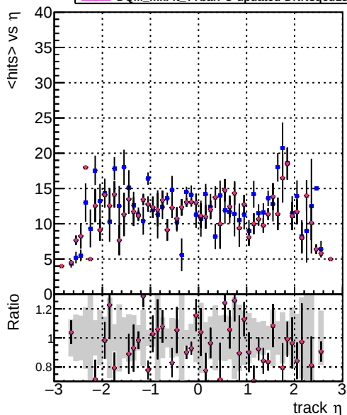
mean hit DQM CKE Tbar DQM mkFit TbarPU-updated DQM mkFit TbarPU-updated-newPLDNN-2 DQM mkFit TbarPU-updated-DNNsqcd13
