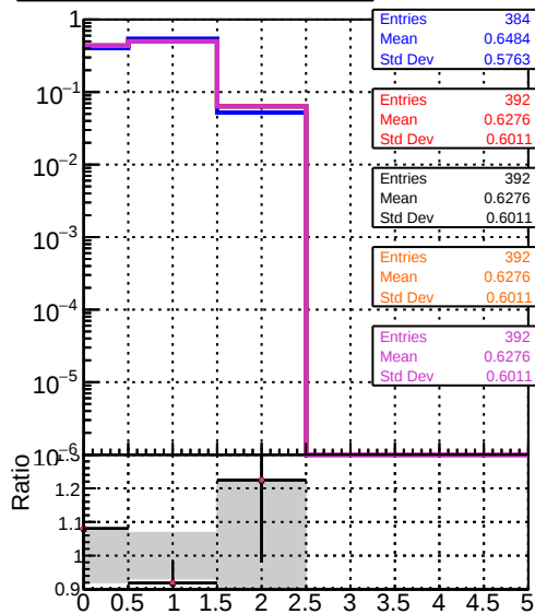
mean hit DQM CKE Tbar DQM mkFit TbarPU-updated DQM mkFit TbarPU-updated-newPLDNN-2 DQM mkFit TbarPU-updated-DNNsqcd13
