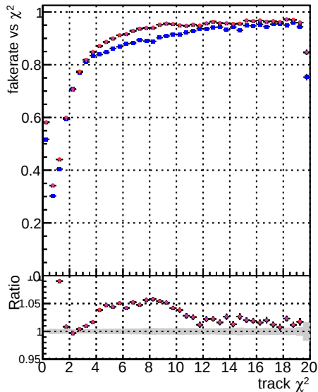
Fake rate vs. DOM CKE TThax TThax updated DOM RL DNN 2
