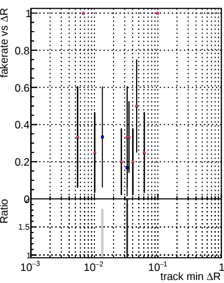
Fake rate vs \Delta R(\text{track, jet}) DQM CKF TTher DQM+PU CKF+PU TTher+PU newPLDNN_2 newPLDNN_2+sqcd13
