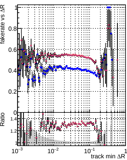
Fake rate vs \Delta R(\text{track, jet}) DQM CKF TTher PU-updated newPLDNN_2 DQM CKF TTher PU-updated newPLDNN_2 DQM CKF TTher PU-updated newPLDNN_2
