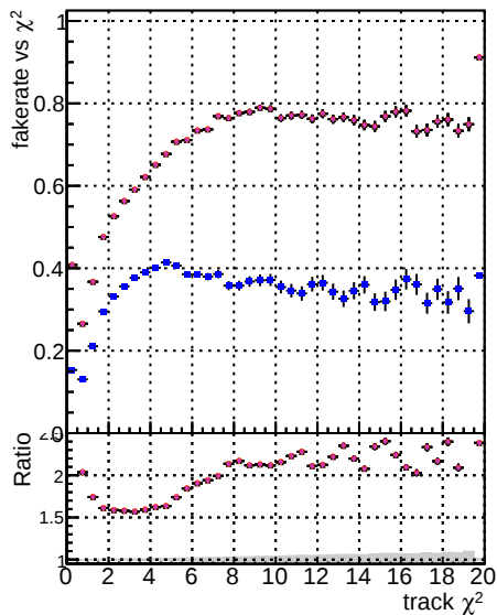
Fake rate vs. DOM GKE TTbar DOM-mkFit TTbar BU-updated newBLDNN-2 DOM-mkFit TTbar BU-updated TTbar DNN-2
