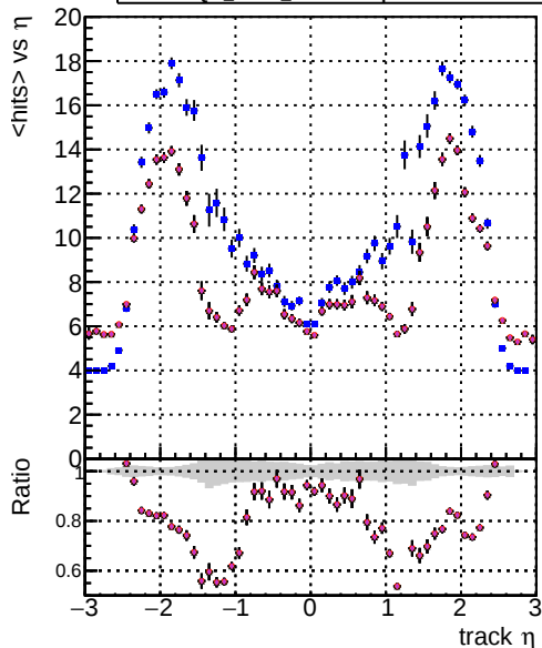
mean hits DOM CKE Ttbar DOM mkFit TtbarPU-updated DOM mkFit TtbarPU-updated-newPLDNN-2 DOM mkFit TtbarPU-updated-TtbarDNN
