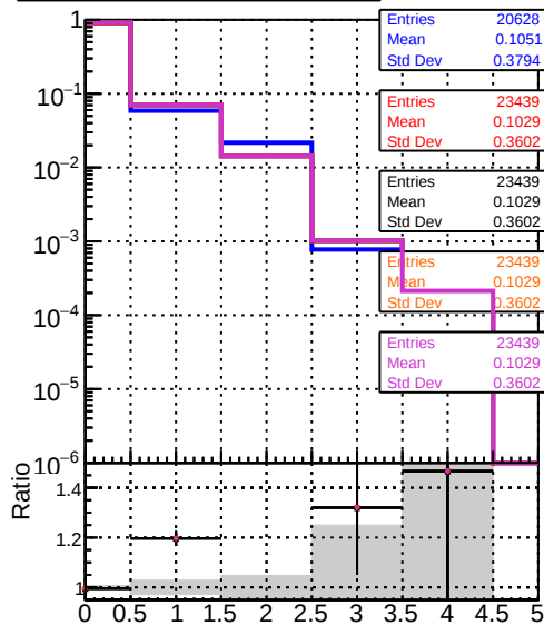
mean hits DOM CKE Ttbar DOM mkFit TtbarPU-updated DOM mkFit TtbarPU-updated-newPLDNN-2 DOM mkFit TtbarPU-updated-TtbarDNN
