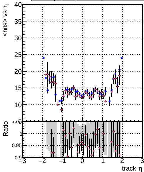
mean hits DOM CKE Ttbar DOM mkFit TtbarPU-updated DOM mkFit TtbarPU-updated-newPLDNN-2 DOM mkFit TtbarPU-updated-newPLDNN DOM mkFit TtbarPU-updated-TtbarDNN
