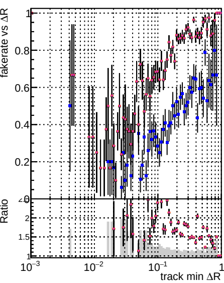
Fake rate vs \Delta R(\text{track, jet}) DQM CKE TTbar PU updated-newBLDNN-2 DQM CKE TTbar PU updated-newBLDNN-2
