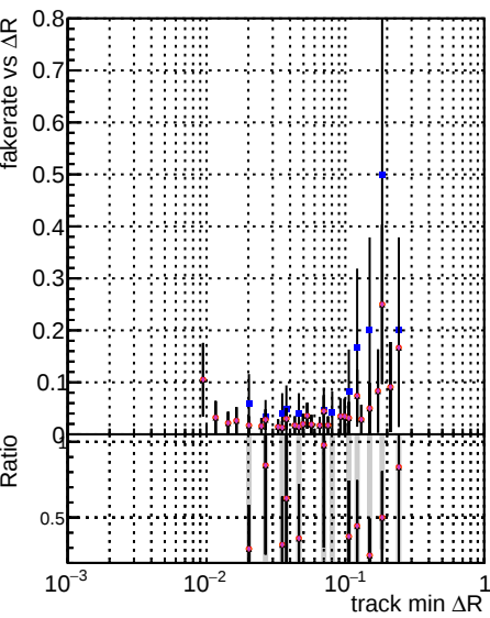
Fake rate vs \Delta R(\text{track, jet}) DQM CKE TThor DQM+PU DQM+PU+updated newBLDNN-2
