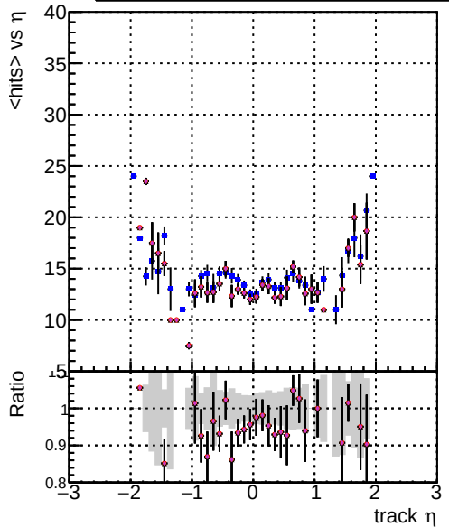
mean hits DOM CKE Ttbar DOM mkFit TtbarPU-updated DOM mkFit TtbarPU-updated-newPLDNN-2 DOM mkFit TtbarPU-updated-TtbarDNN DOM mkFit TtbarPU-updated-TtbarDNN
