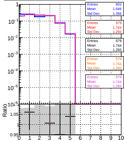
mean hit DOM CKE Ttbar DOM mkFit TtbarPU-updated DOM mkFit TtbarPU-updated-newPLDNN DOM mkFit TtbarPU-updated-newPLDNN-2
