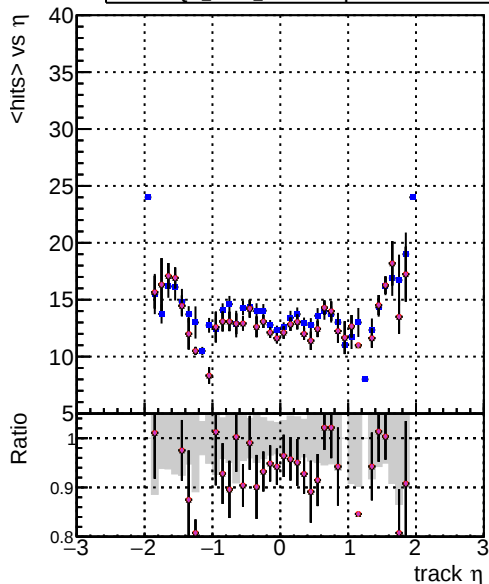
mean hit DOM CKE Ttbar DOM mkFit TtbarPU-updated DOM mkFit TtbarPU-updated-newPLDNN-2 DOM mkFit TtbarPU-updated-TtbarDNN
