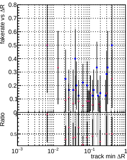
Fake rate vs \Delta R(\text{track, jet}) DQM CKF TThor PU PU-updated newPLDNN-2
