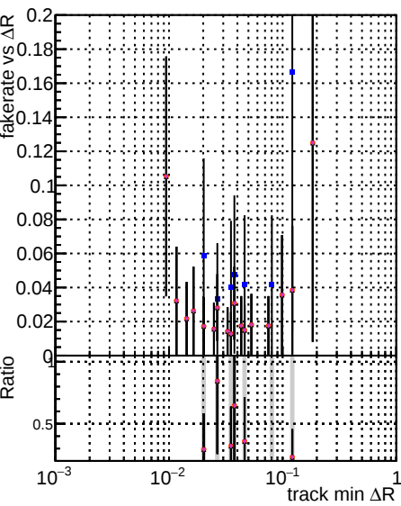
Fake rate vs \Delta R(\text{track, jet}) DQM CKE TThor TThor PU-updated newBLDNN-2 DQM CKE TThor TThor PU-updated newBLDNN-2
