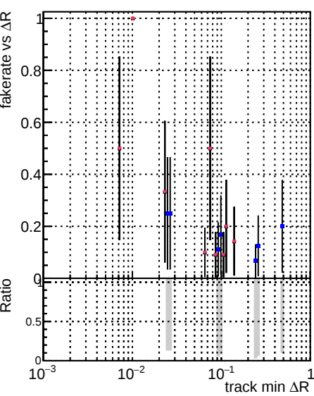
Fake rate vs \Delta R(\text{track}, \text{jet}) DQM CKF TThor DQM+CKF CKF+TThor TThor+DQM DQM+CKF+TThor DQM+CKF+TThor+newBLDNN-2 DQM+CKF+TThor+newBLDNN-2
