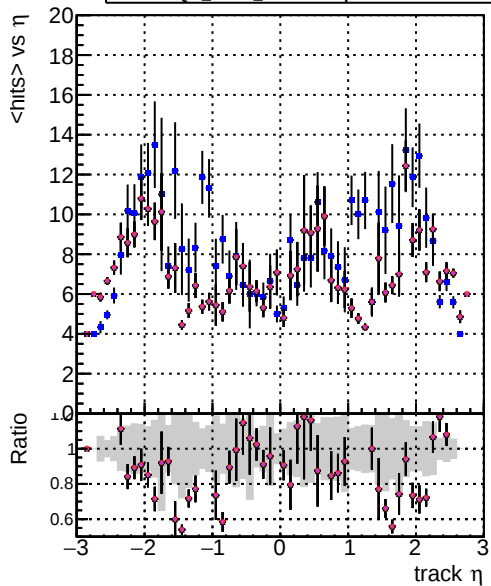
mean hit DQM CKE Tbar DQM mkFit TbarPU-updated DQM mkFit TbarPU-updated-newPLDNN-2 DQM mkFit TbarPU-updated-TTbarDNN
