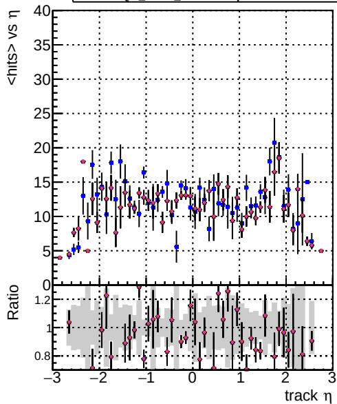
mean hit DQM CKE Ttbar DQM mkFit TtbarPU-updated DQM mkFit TtbarPU-updated-newPLDNN-2 DQM mkFit TtbarPU-updated-TtbarDNN
