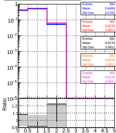
mean hit DQM CKE Ttbar DQM mkFit TtbarPU-updated DQM mkFit TtbarPU-updated-newPLDNN-2 DQM mkFit TtbarPU-updated-TtbarDNN
