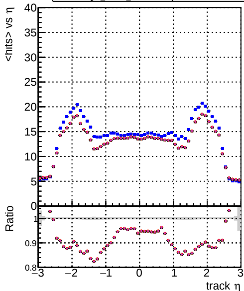
mean hit DOM CKE Ttbar DOM mkFit TtbarPU-updated DOM mkFit TtbarPU-updated-newPLDNN DOM mkFit TtbarPU-updated-newPLDNN-2
