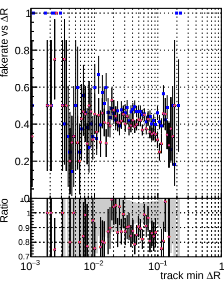
Fake rate vs \Delta R(\text{track, jet}) DQM CKF Tthor Tthor PU-updated newBLDNN-2 DQM CKF Tthor Tthor PU-updated newBLDNN-2
