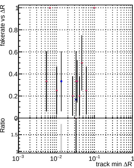
Fake rate vs \Delta R(\text{track, jet}) DQM CKF TThor DQM+PU CKF+PU TThor+PU DQM+PU+updated-new DQM+PU+updated-new+BLDNN-2
