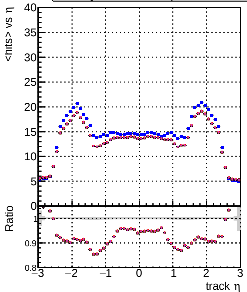
mean hit DOM CKE Ttbar DOM mkFit TtbarPU-updated DOM mkFit TtbarPU-updated-newPLDNN DOM mkFit TtbarPU-updated-newPLDNN-2 DOM mkFit TtbarPU-updated-TtbarDNN
