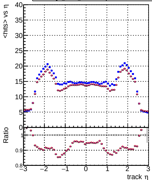
mean hit DOM CKE Ttbar DOM mkFit TtbarPU-updated DOM mkFit TtbarPU-updated-newPLDNN DOM mkFit TtbarPU-updated-TtbarDNN-2
