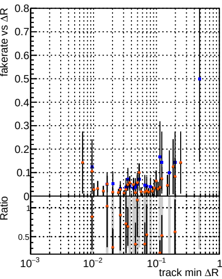
Fake rate vs \Delta R(\text{track, jet}) Legend: DOM, CKE, Ttbar, PU-updated, mktfit, TtbarPU-updated, PLBNN-2, mktfit, TtbarPU-updated-new, PLBNN-2
