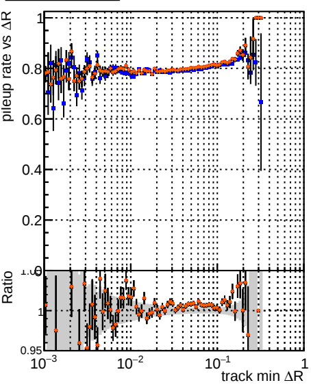
DOM CKE Ttbar mkrfit TtbarPU-updated mkrfitPU-updated-newPLBNN-2
