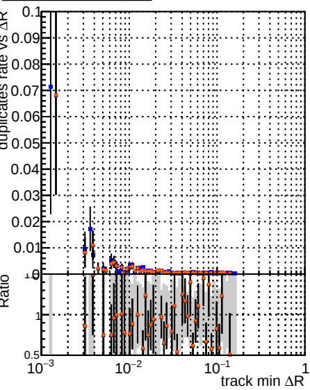
DOM CKE Ttbar mkrfit TtbarPU-updated mkrfitPU-updated-newPLBNN-2
