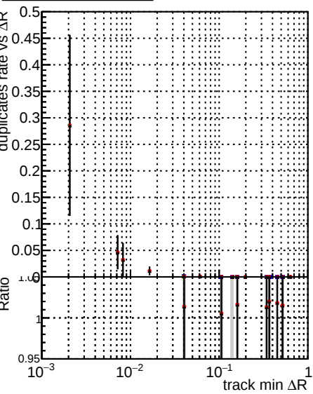
Legend: DOM_CKF_softQCD, DOM_mkFit_SoftQCD-updated1, DOM_mkFit_SoftQCD-updated1-newPLDNN
