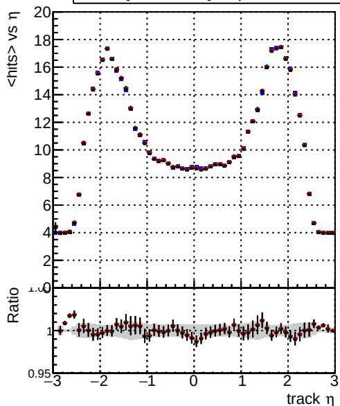
mean hits vs \eta DQM_CKF_softQCD DQM_mkFit_SoftQCD-updated1 DQM_mkFit_SoftQCD-updated1-newPLDNN
