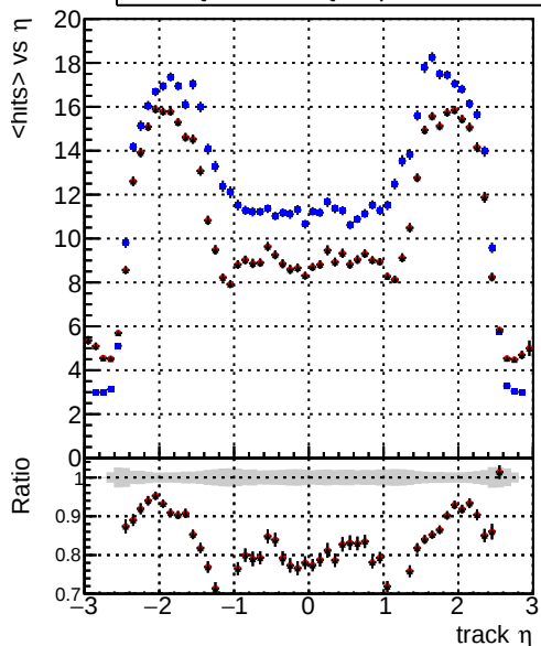
mean hits — DQM_CKF_softQCD — DQM_mkFit_SoftQCD-updated1 — DQM_mkFit_SoftQCD-updated1-newPLDNN
