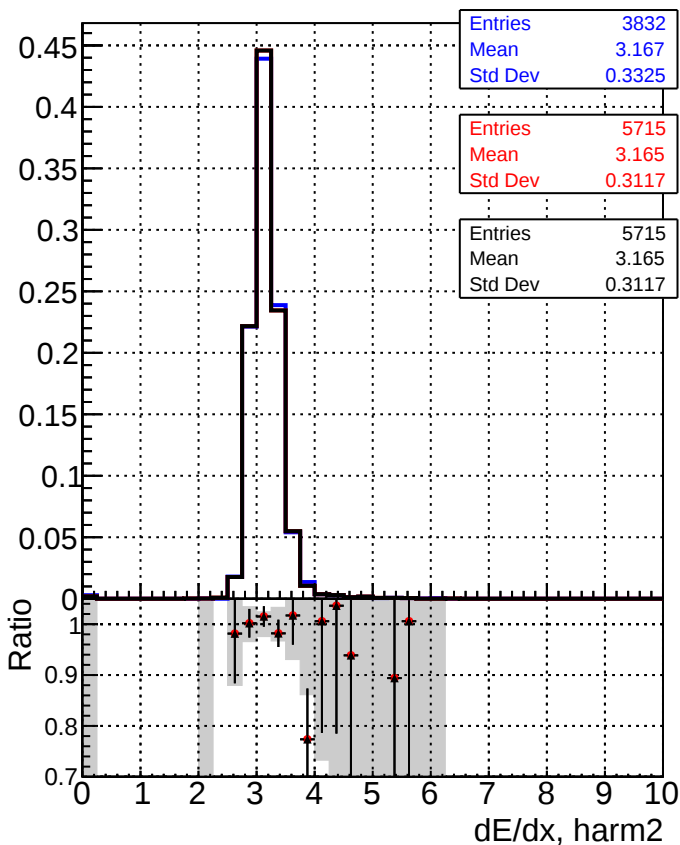
—■— DQM_CKF_softQCD —●— DQM_mkFit_SoftQCD-updated1 —▲— DQM_mkFit_SoftQCD-updated1-newPLDNN
