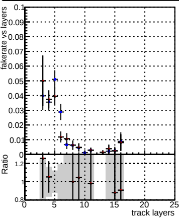
Fake rate vs hit DQM_CKF_softQCD DQM_mkFit_SoftQCD-updated1 DQM_mkFit_SoftQCD-updated1-newPLDNN
