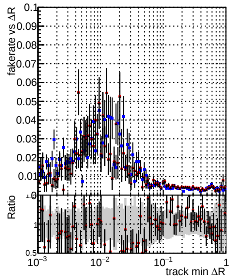
—●— DQM_CKF_softQCD —●— DQM_mkFit_SoftQCD-updated1 —●— DQM_mkFit_SoftQCD-updated1-newPLDNN
