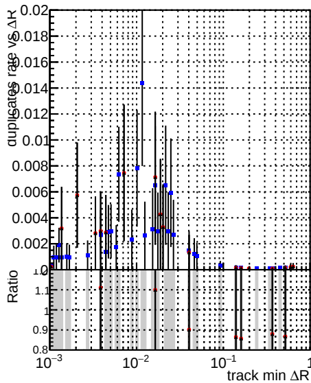
—●— DQM_CKF_softQCD —●— DQM_mkFit_SoftQCD-updated1 —●— DQM_mkFit_SoftQCD-updated1-newPLDNN
