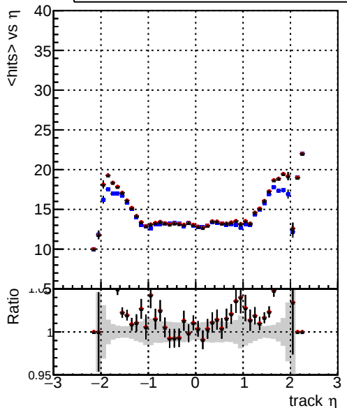
mean hit — DQM_CKF_softQCD — DQM_mkFit_SoftQCD-updated1 — DQM_mkFit_SoftQCD-updated1-newPLDNN
