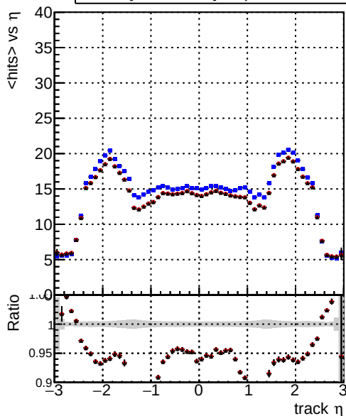
mean hit — DQM_CKF_softQCD — DQM_mkFit_SoftQCD-updated1 — DQM_mkFit_SoftQCD-updated1-newPLDNN
