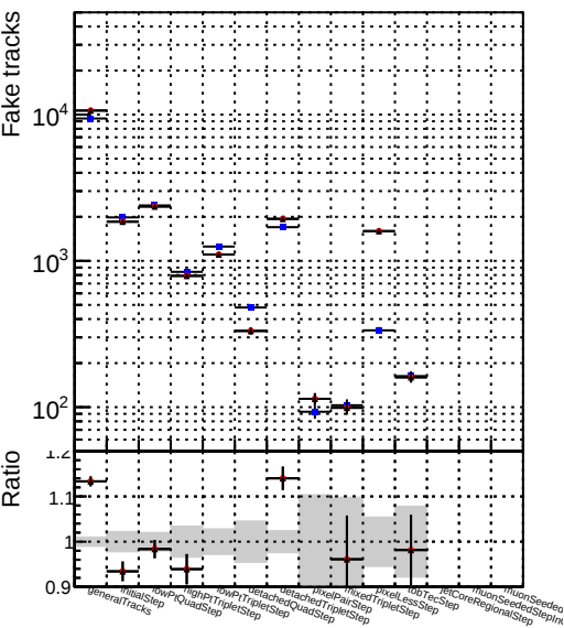
Number DQM_mkFit_SoftQCD-updated DQM_mkFit_SoftQCD-DNNalliters
