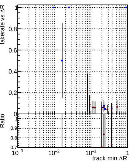
Fake rate vs \Delta R(\text{track, jet}) DQM_CKF_softQCD DQM_mkFit_SoftQCD-updated DQM_mkFit_SoftQCD-DNNalliters
