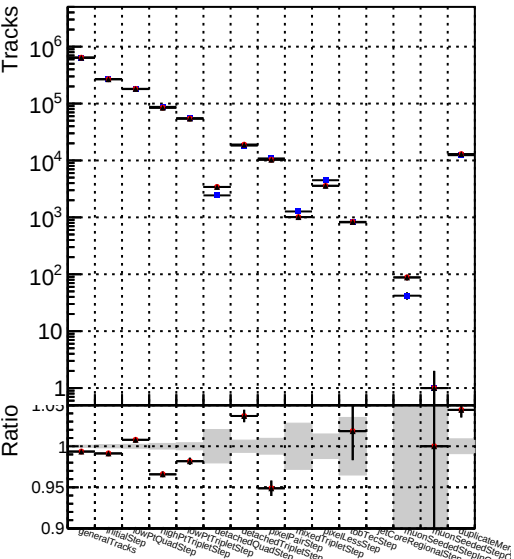
Number —■— DQM_CKF_softQCD —●— DQM_mkFit_SoftQCD-updated —▲— DQM_mkFit_SoftQCD-DNNalliters
