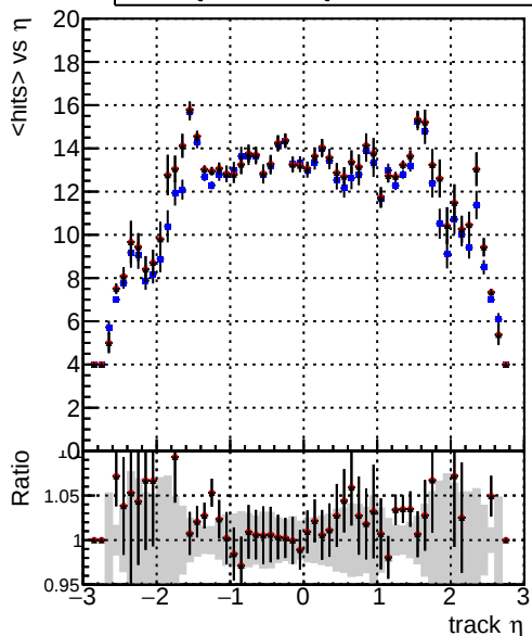
mean hit — DQM_CKF_softQCD — DQM_mkFit_SoftQCD-updated — DQM_mkFit_SoftQCD-DNNalliters
